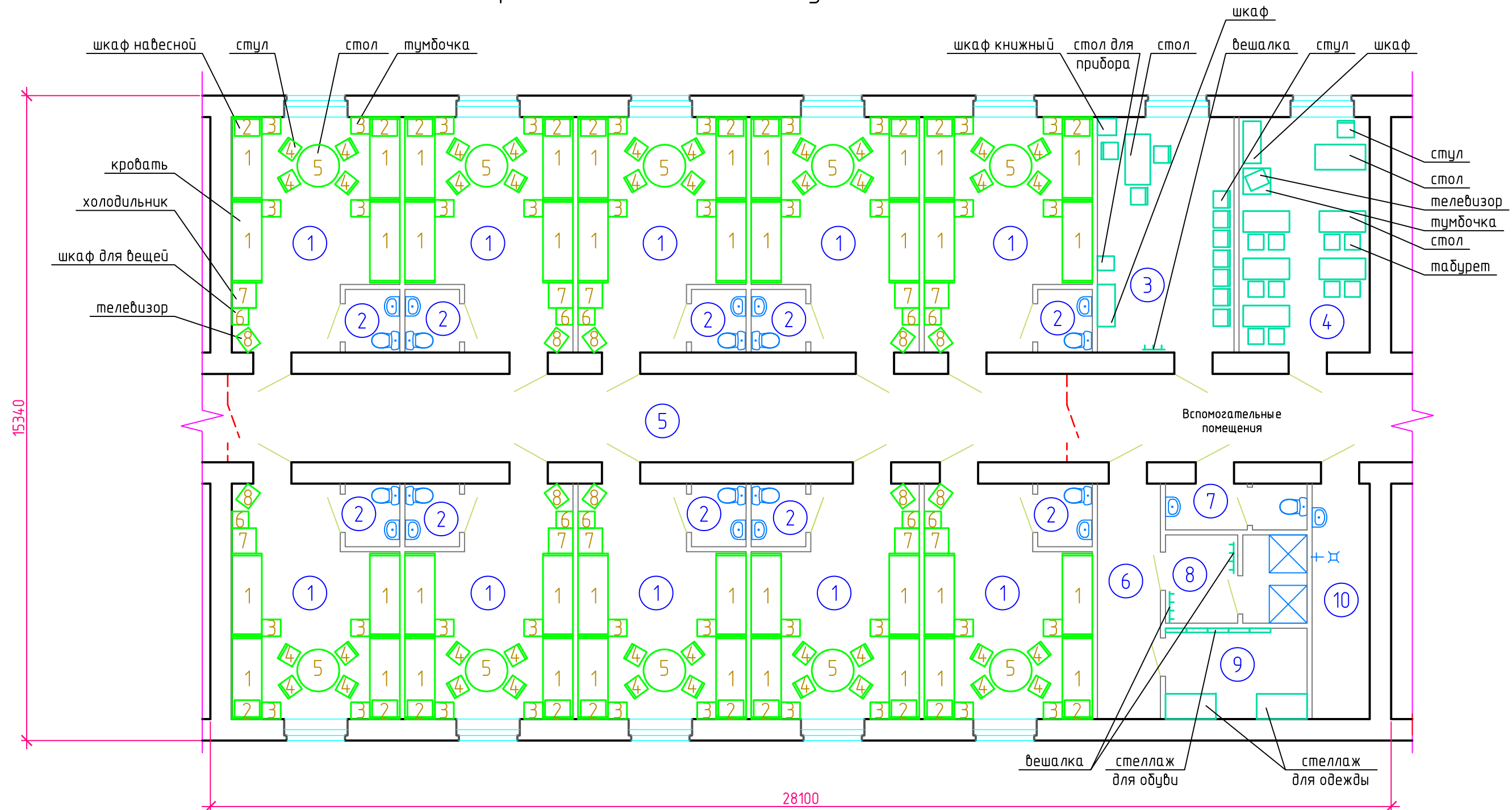
Экспликация помещений (начало)
