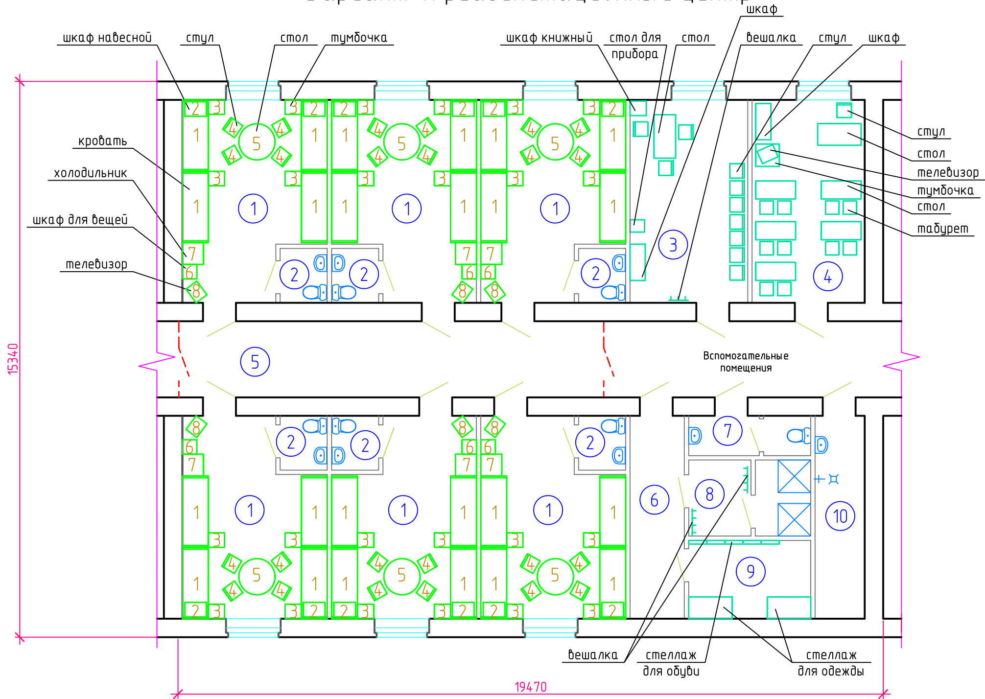
Экспликация помещений (начало)
